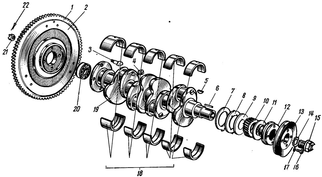
Рис. 6. Коленчатый вал и маховик Рис. 6. Колянов вал и маховик Výkres 6. Klikový hřídel a setrvačnick 6. ábra. Forgattyústengely és lendkerék Rys. 6. Wał korbowy i koło zamachowe
